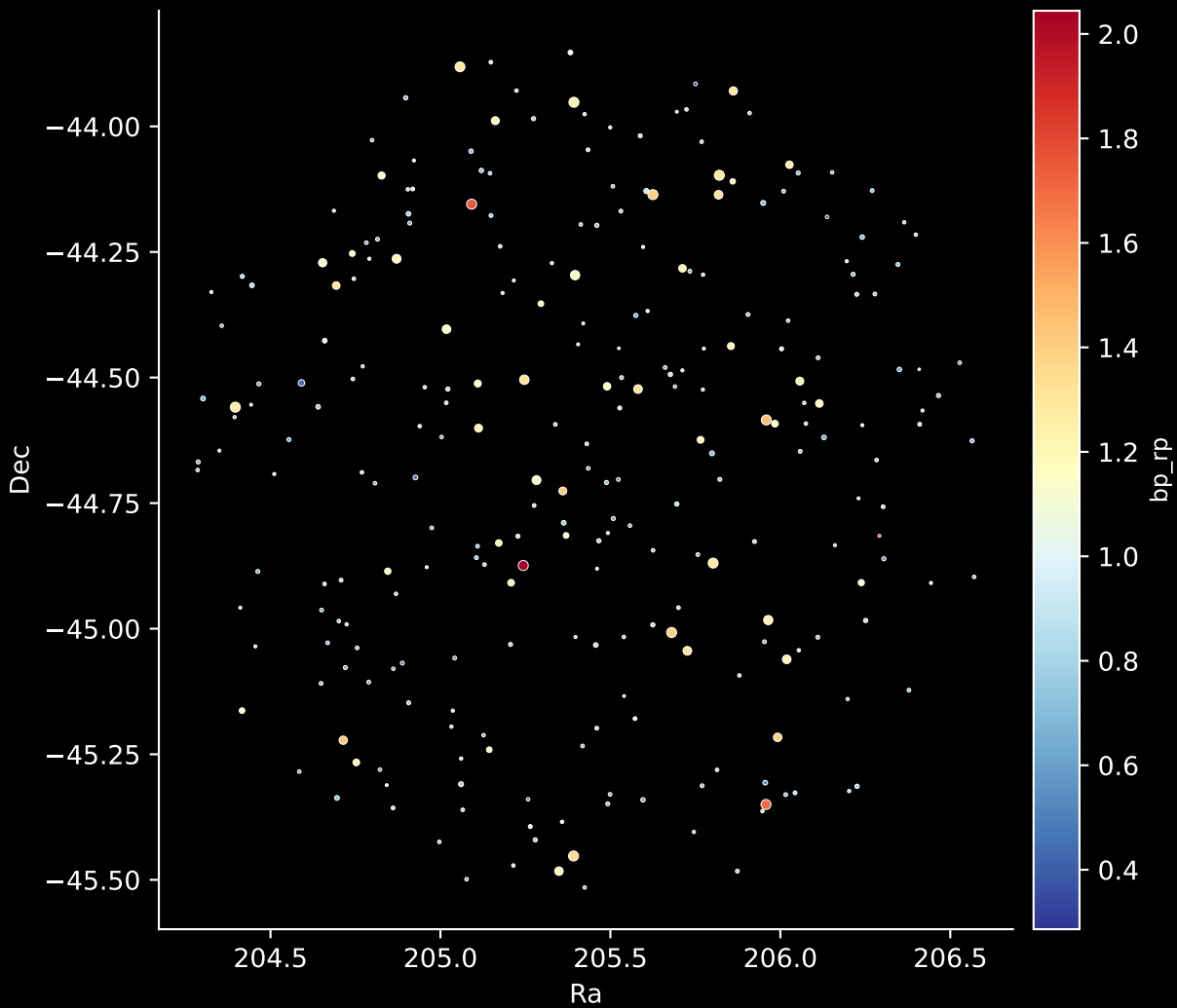
GALAH DR4 Field: [2600] Stars: 261
