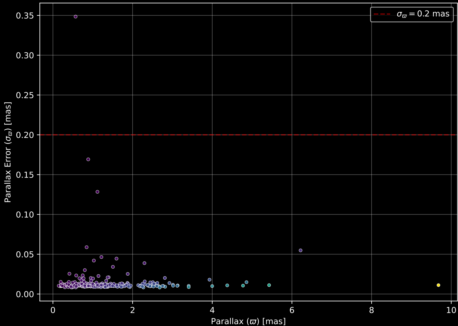
GALAH DR4 Field: [2600] Parallax Quality (n= 261)
