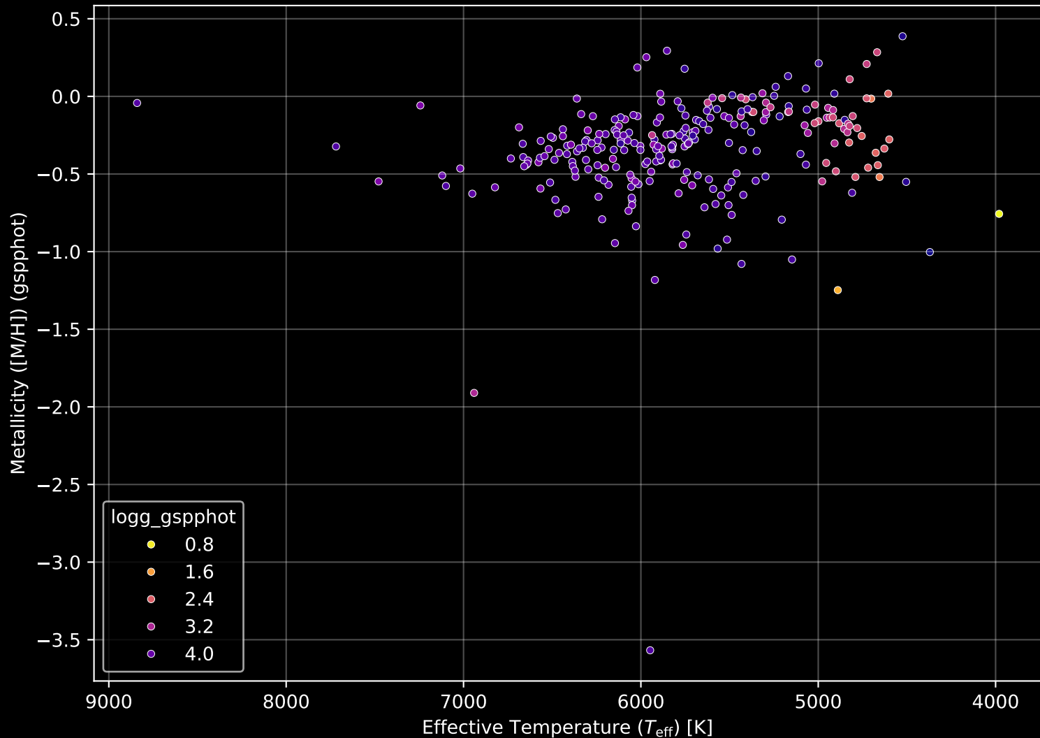
GALAH DR4 Field: [2600] Stellar Population Parameters (n= 261)
