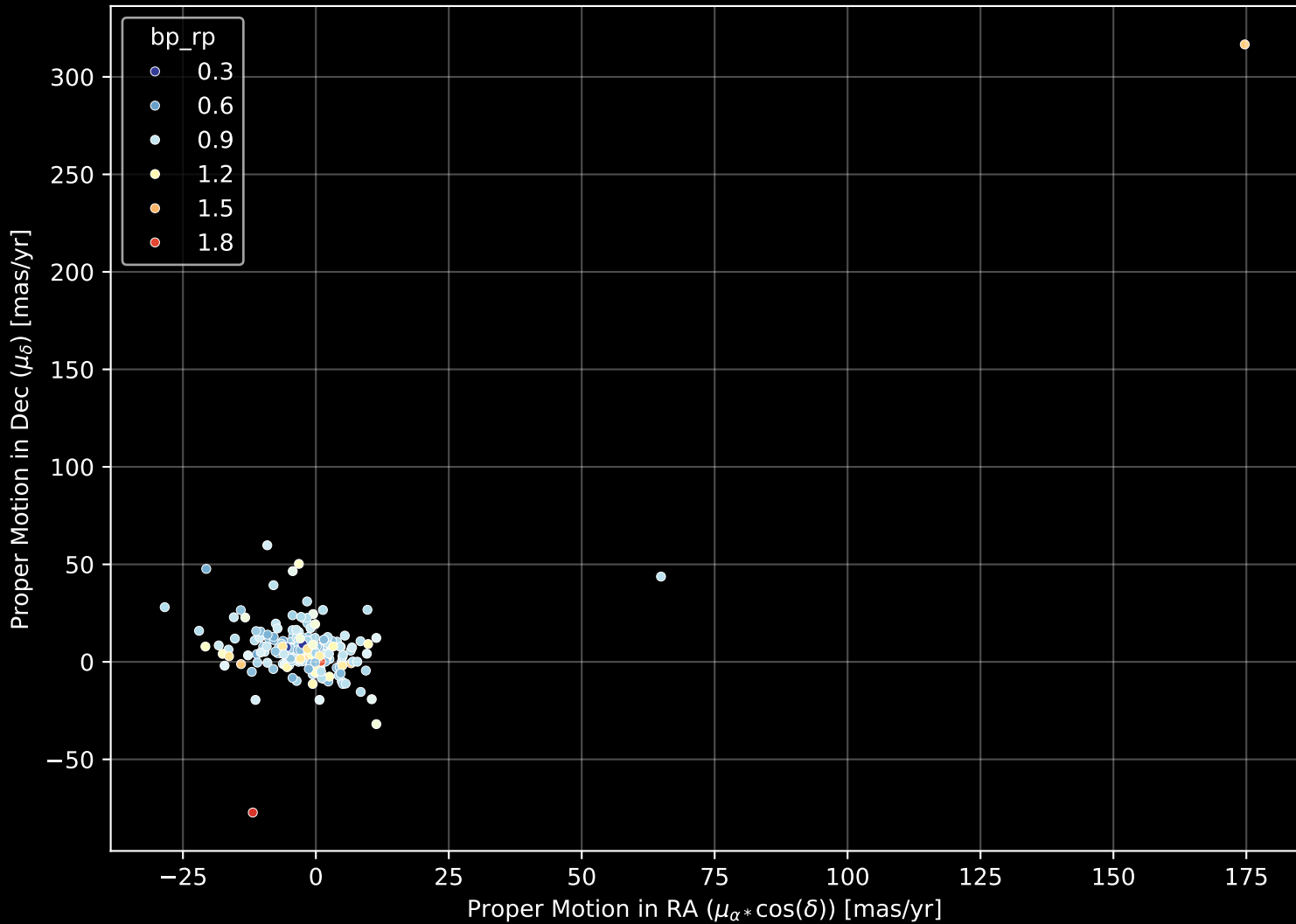
GALAH DR4 Field: [2600] Proper Motion Diagram (n= 261)
