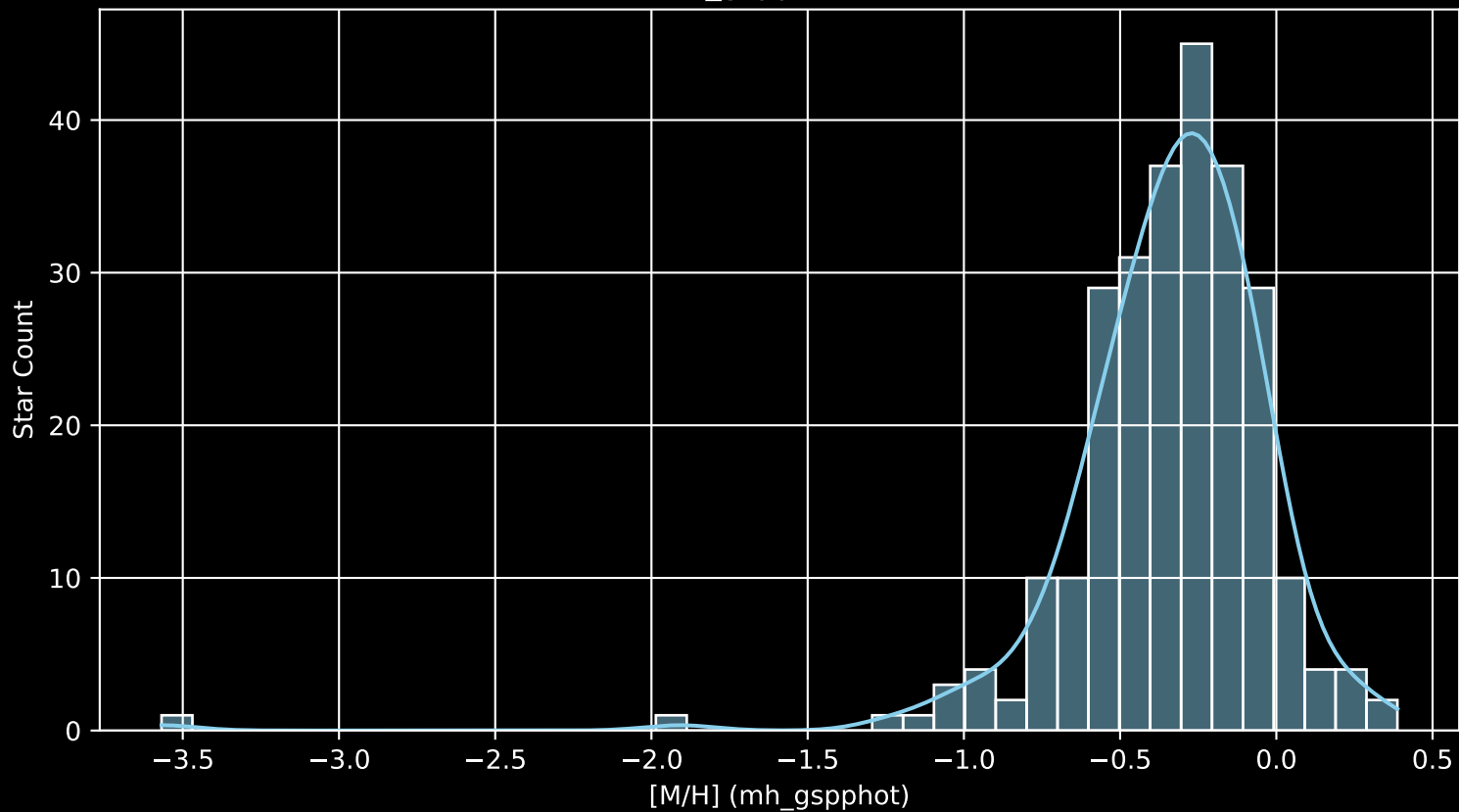
GALAH DR4 Field: [2600] [M/H] (mh_gspphot) (n= 261)
